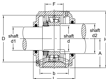
Type:SNZ300
