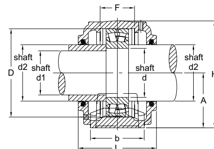
Type:SN300
