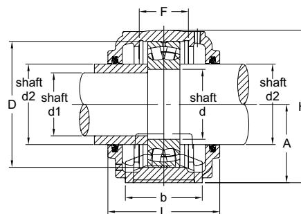
Type:SN200
